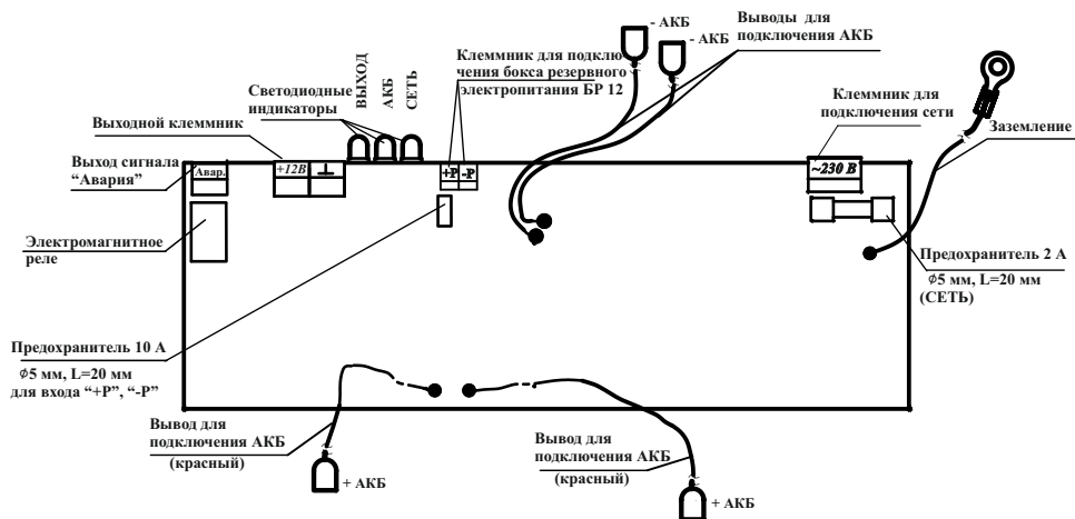
Рисунок 1 – Плата источника
